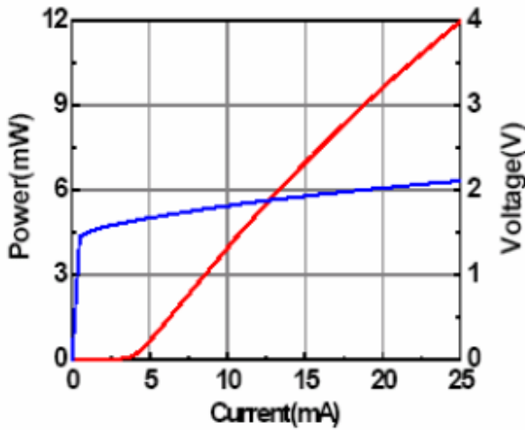
LIV Curve
