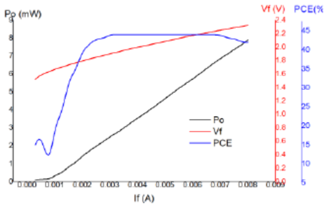
LIV Curve
