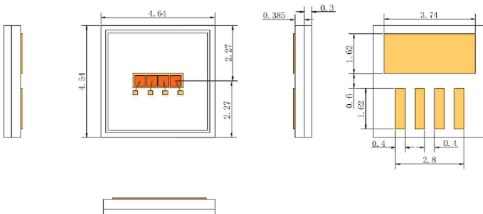
1x4 Array
